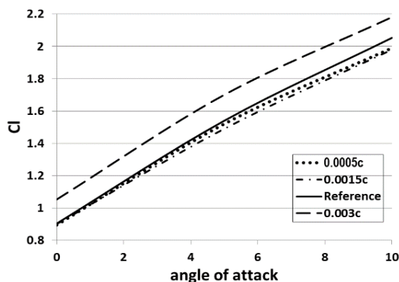
شکل ۵ مقادیر ضریب برآ در زاویه فلپ ۱۰ درجه
