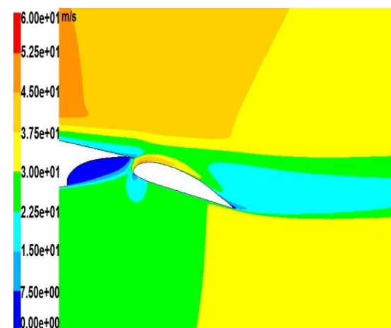
شکل ۱۸ کانتور سرعت با اوورلپ 0/0025C در زاویه فلپ و حمله 10 درجه
