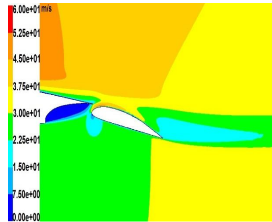
شکل ۱۷ کانتور سرعت با اوورلپ 0/003C در زاویه فلپ و حمله 10 درجه
