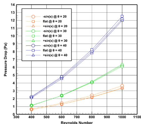
شکل ۱۱ تغییرات افت فشار در زوایای حمله مختلف
