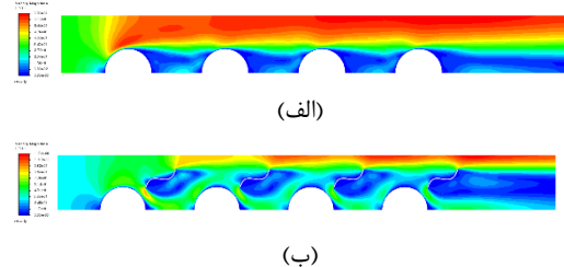
شکل ۱۵ کانتورهای مربوط به میدان سرعت (الف) بدون حضور مولد گردابه (ب) با حضور مولد گردابه سینوسی
