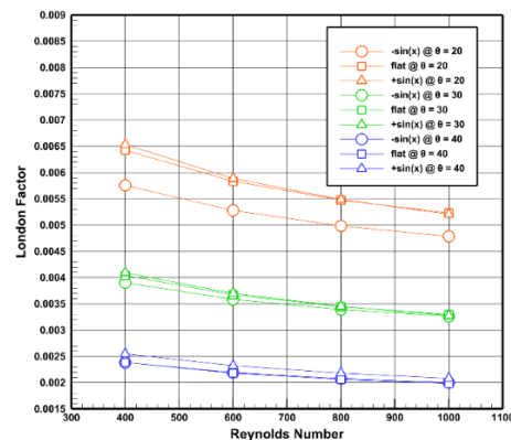
شکل ۱۳ نمودار ضریب لندن برحسب عدد رینولدز
