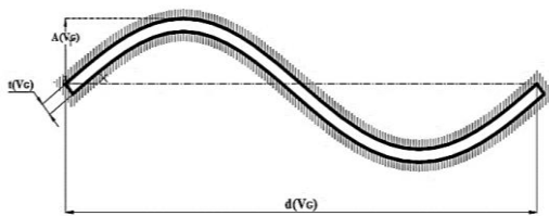
شکل ۴ مشخصات ابعادی مولدهای گردابه با ضابطه موج سینوسی
