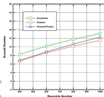
شکل ۷ راستی آزمایشی مقاله حاضر در اعداد رینولدز مختلف
