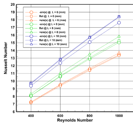
شکل ۱۰ تغییرات میانگین عدد نوسلت در طول‌های مختلف
