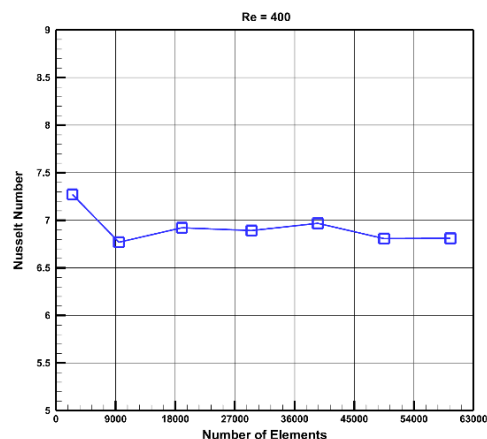
شکل ۵ نمودار تغییرات عدد نوسلت متوسط در تعداد المان‌های مختلف از شبکه‌بندی در عدد رینولدز ۴۰۰
