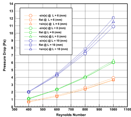
شکل ۱۲ تغییرات افت فشار در طول‌های مختلف
