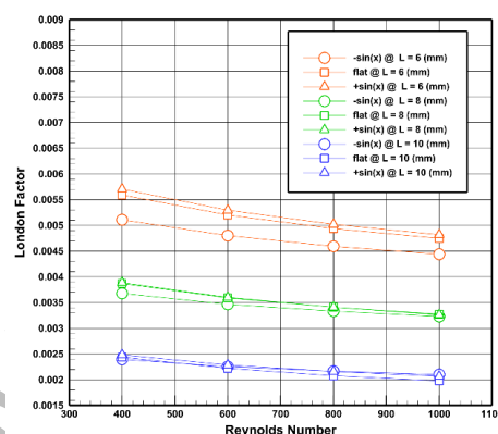
شکل ۱۴ نمودار تغییرات ضریب لندن در رینولدزهای مختلف
