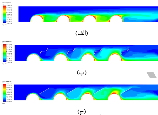
شکل ۱۶ کانتورهای میدان دما (الف) بدون حضور مولد گردابه (ب) با حضور مولد گردابه سینوسی در زاویه حمله ۴۰ درجه (ج) با حضور مولد گردابه تخت در طول ۱۰ میلی‌متری.
