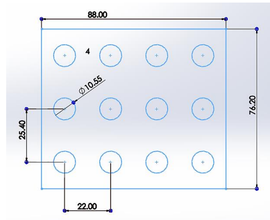
شکل ۲ ابعاد میدل حرارتی از نمای بالا به میلی‌متر
