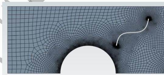
شکل ۶ شبکه بندی منتخب با تعداد ۱۹۰۰۰ المان
