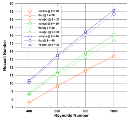
شکل ۹ تغییرات میانگین عدد نوسلت در زوایای حمله مختلف
