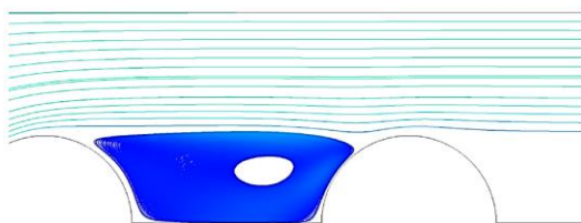
شکل ۸ ناحیه برگشت جریان میان دو لوله همجوار
